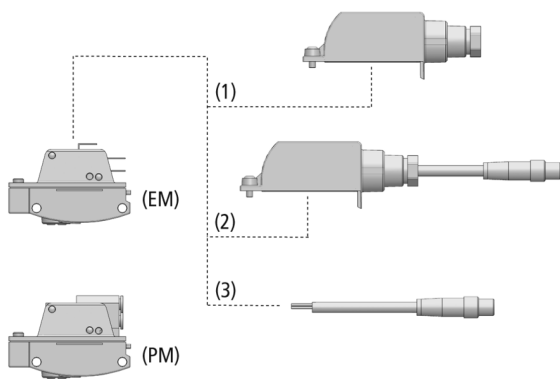
Diseño del sistema Vacuestatos VS-V-PM/EM-ST
